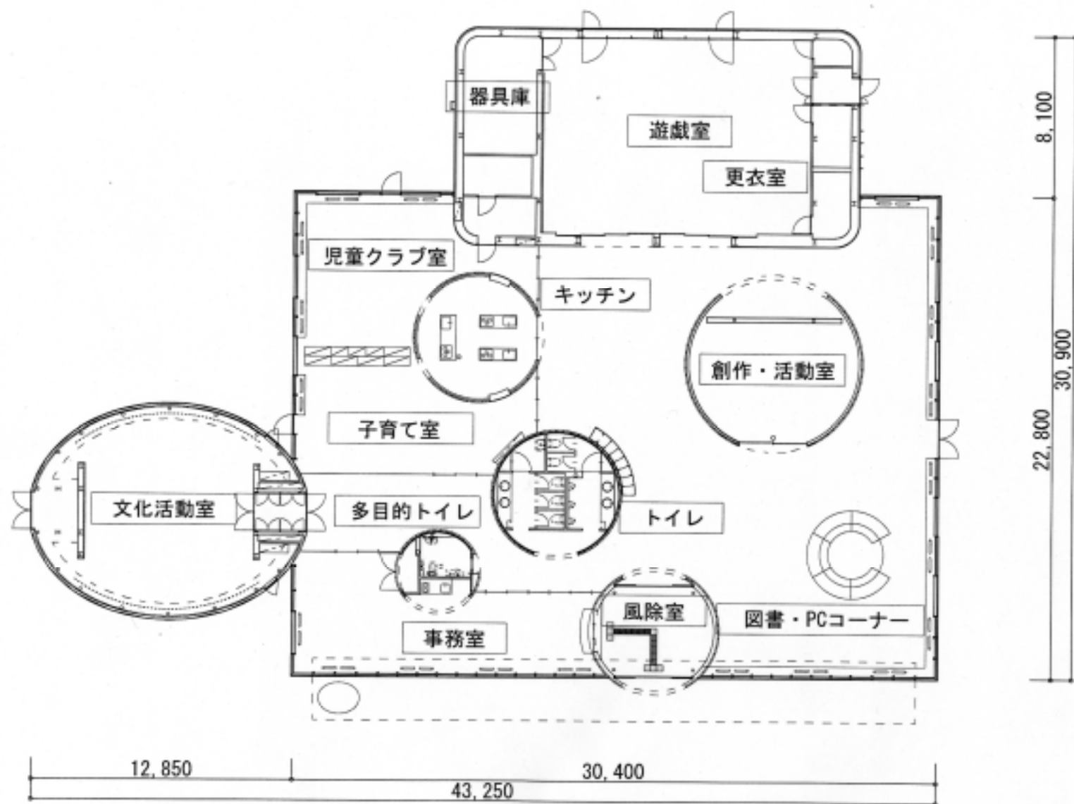
平面図
