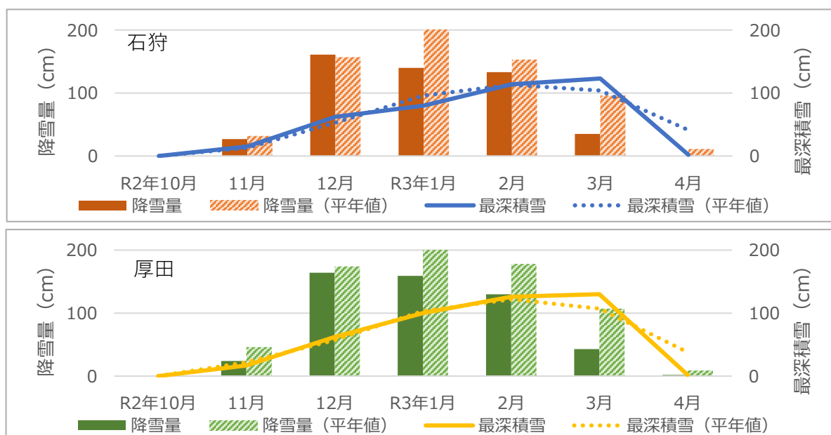
図 6-18 地区別の月別降雪量及び最深積雪
