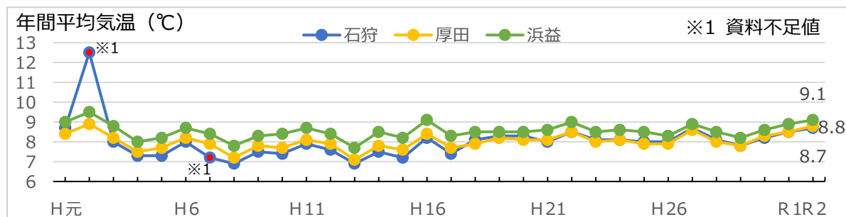
図 6-13 石狩地区、厚田地区、浜益地区の年平均気温
