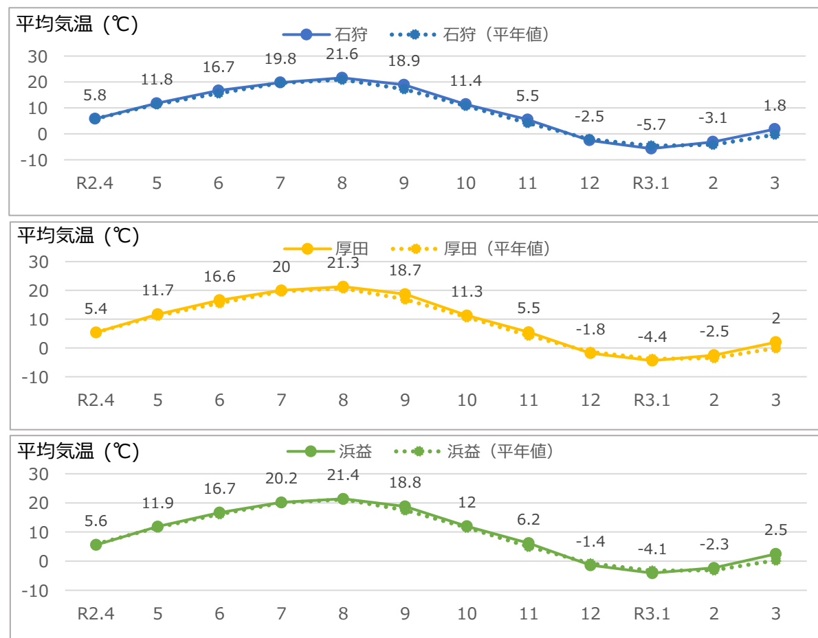
図 6-14 地区別の令和2年度月別平均気温
