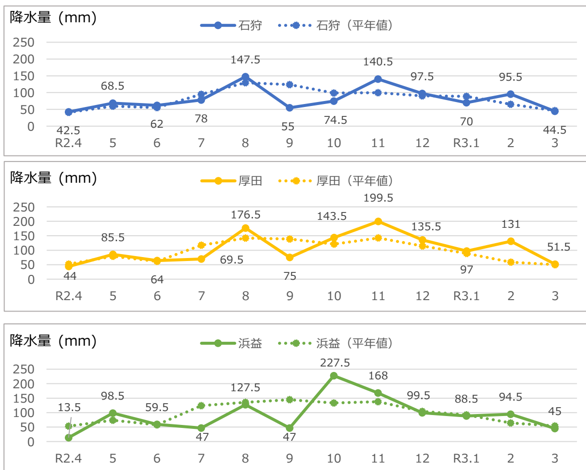
図 6-16 地区別の令和2年度月別降水量
