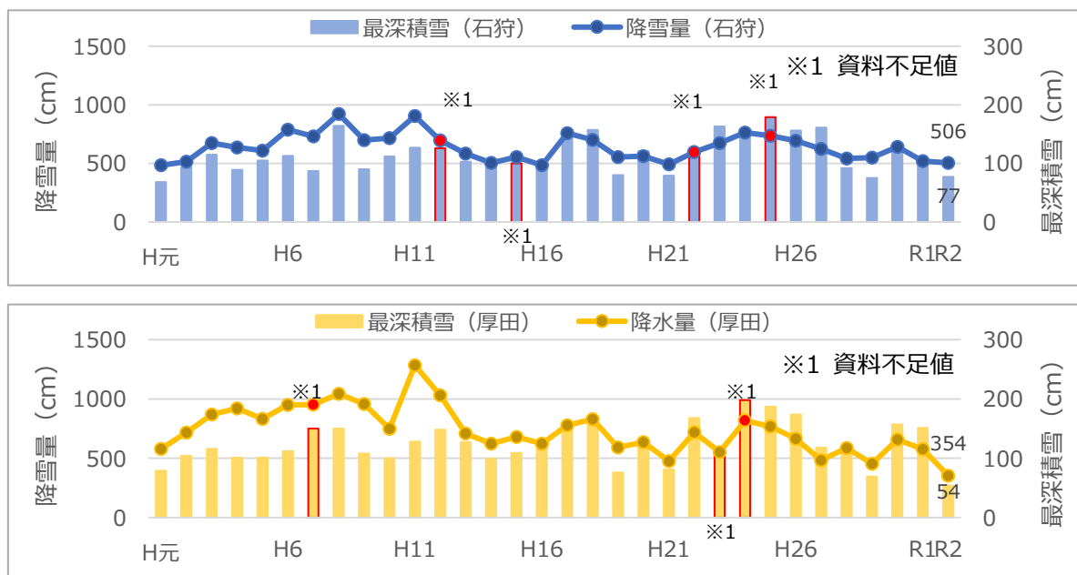
図 6-17 地区別の年別降雪量及び最深積雪
