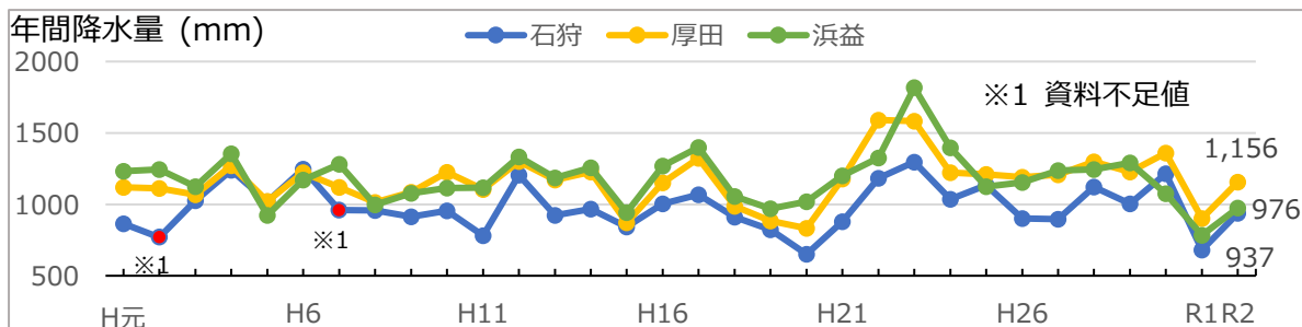
図 6-15 石狩地区、厚田地区、浜益地区の年間降水量
