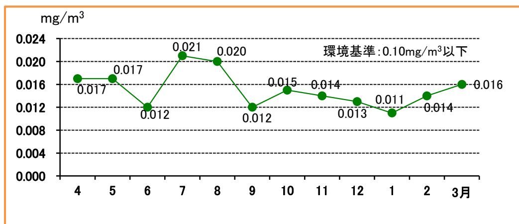
図 3-6 平成 27 年度 浮遊粒子状物質の経月変化（月平均値）
