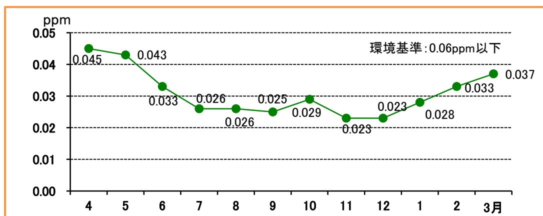
図3-4 平成27年度 光化学オキシダントの経月変化（月平均値）
