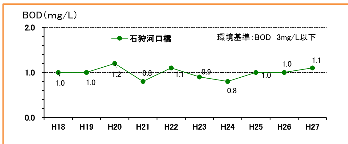
図3-9 平成27年度 石狩川のBOD 経年変化（75%値 ※3 ）
