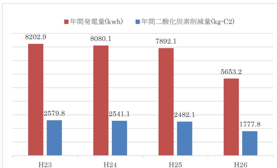
図7-5 市役所庁舎太陽光発電システムの年間発電量および年間二酸化炭素削減量の推移 (市環境政策課調べ)
