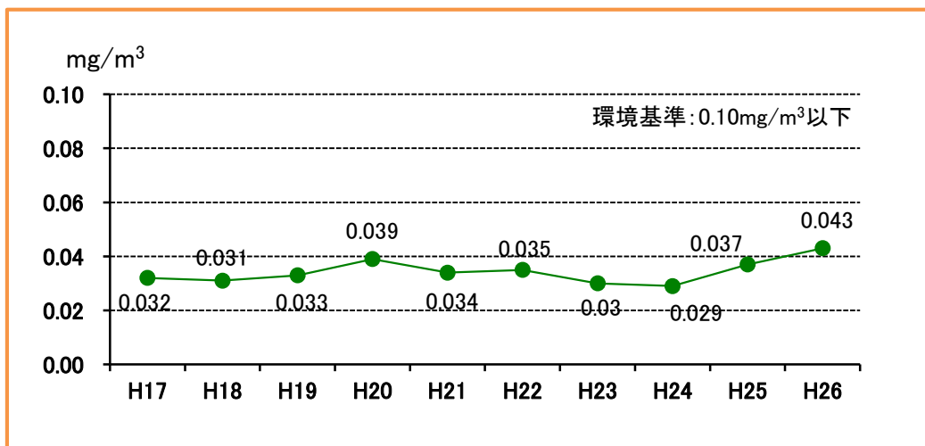
図 3-7 浮遊粒子状物質の経年変化（日平均値の 2%除外値 ※4 ）
