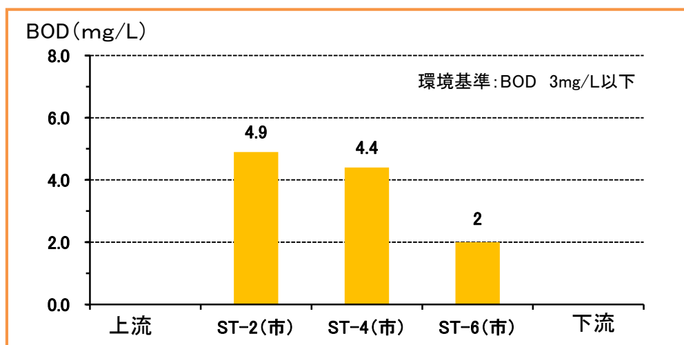
図3-16 平成26年度 荻戸川のBOD調査地点別変化(75%値)
