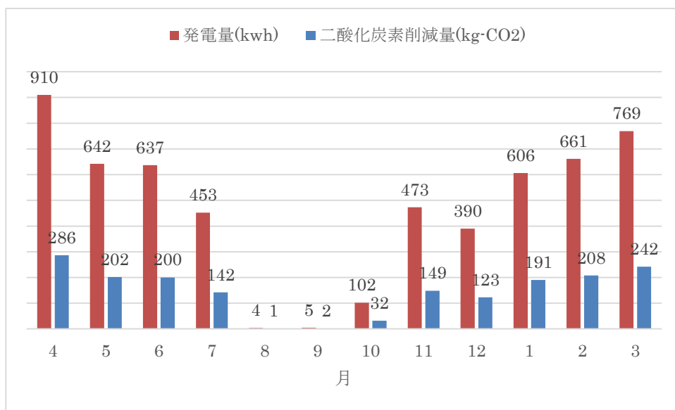
図7-4 平成26年度市役所庁舎太陽光発電システムの発電量および二酸化炭素削減量 (市環境政策課調べ)
