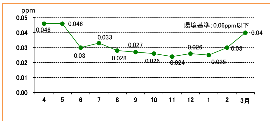
図3-4 平成26年度 光化学オキシダントの経月変化（月平均値）
