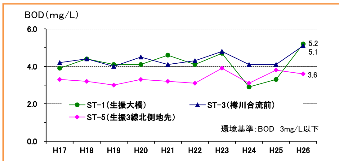
図3-15 茨戸川のBOD経年変化（75%値）
