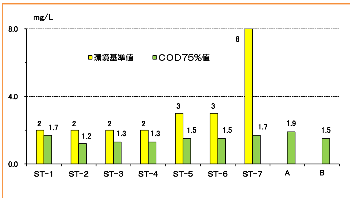
図3-13 平成26年度 石狩海域のCOD調査結果
