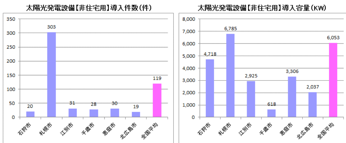
図 7－6 太陽光発電設備導入件数・導入容量【非住宅用】
