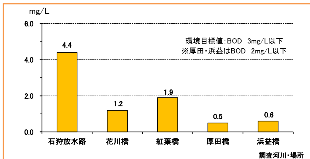
図3-18 平成26年度 中小河川のBOD調査結果(75%値)
