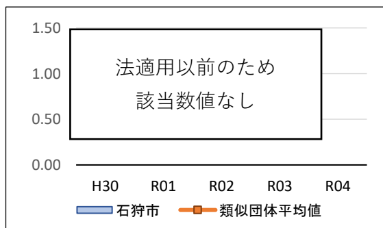
図-17 流動比率（％）
