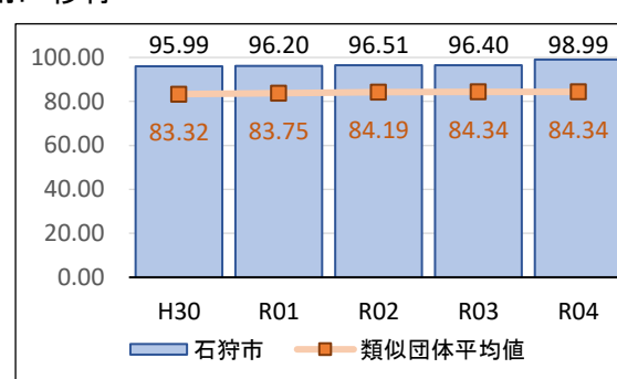
図-31 水洗化率(%)
