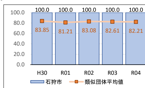
図-32 水洗化率(%)
