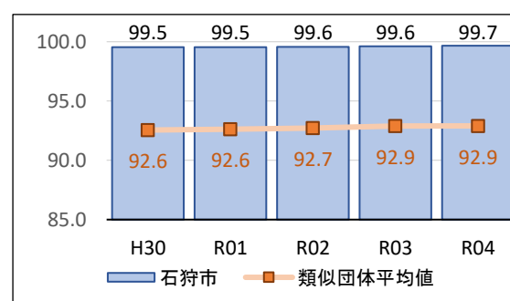
図-30 水洗化率(%)
