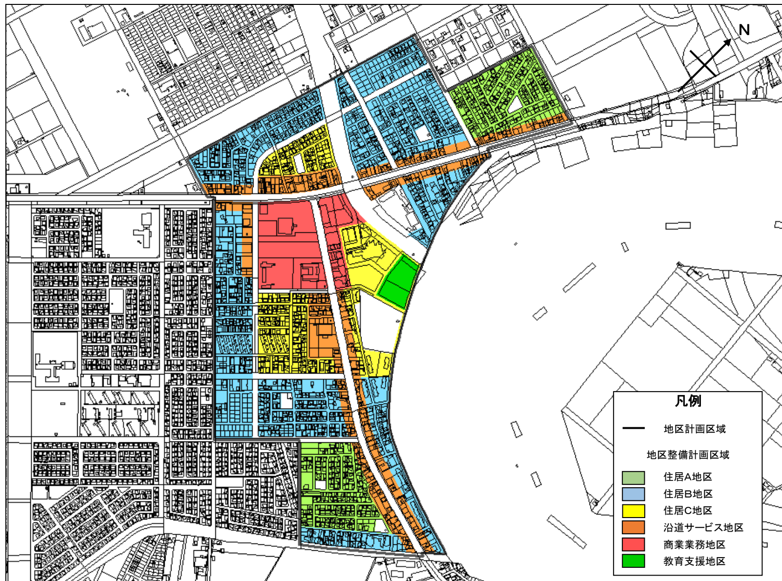
札幌圏都市計画地区計画(石狩都心地区) 計画図
