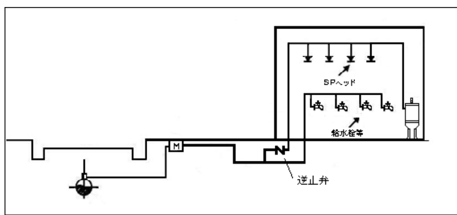
図－4 湿式方式
