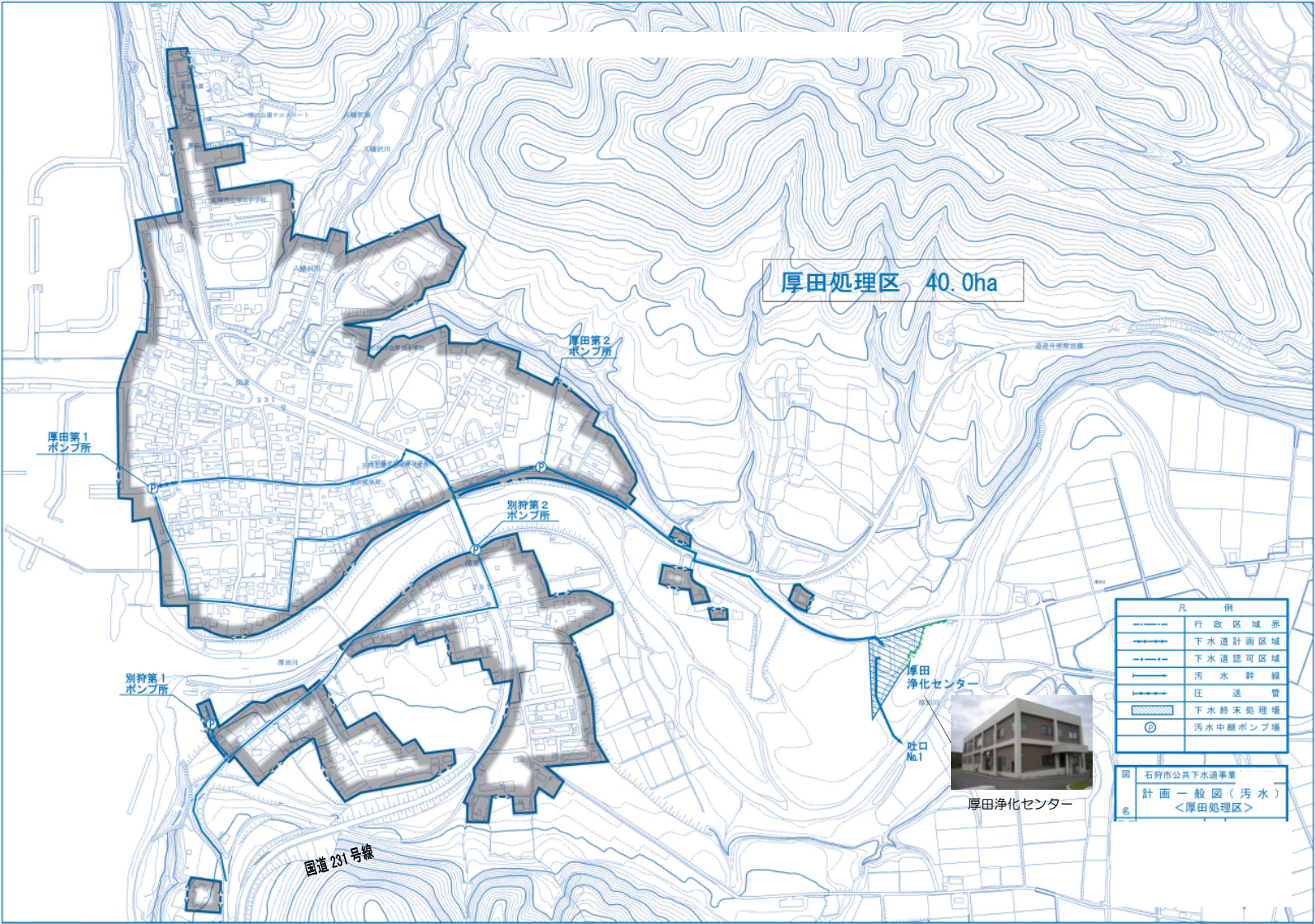
図 2-4 汚水施設(厚田処理区)
