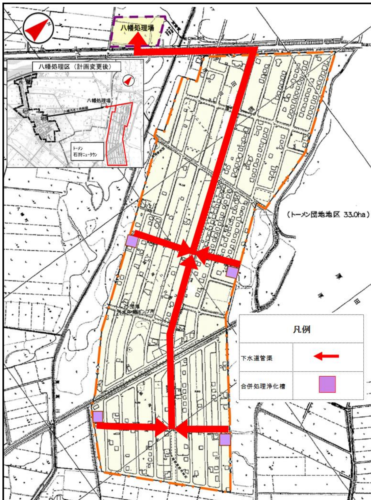
トーマン石狩ニュータウン下水道施設整備予定図
