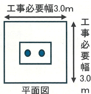
参考図①(設置スペース5人槽)
