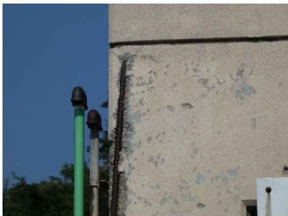
外壁の鉄筋露出〔生振小〕
