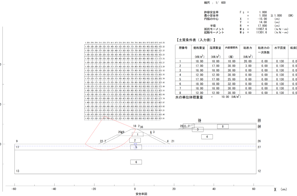
図 11-8 安定解析結果（嵩上げ（軽微変更届出） 旧基準 地震時）
