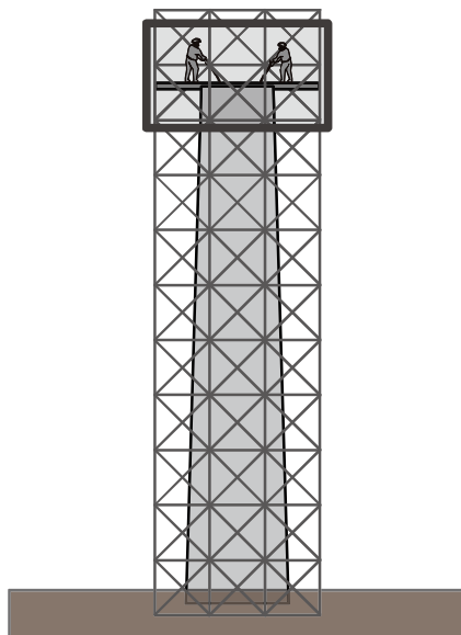
図 4-45 人力ブレーカー解体工法の概念図
