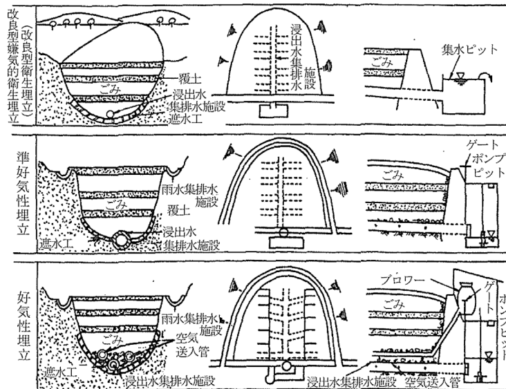
図 4-29 埋立構造概念図
