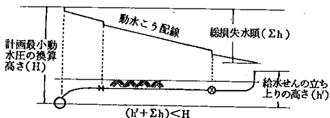
図 2-2 水頭変化曲線図
