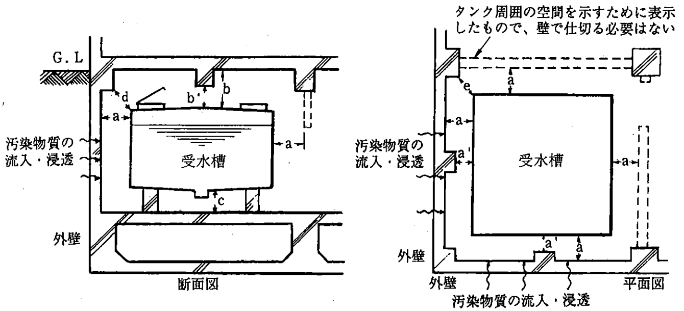
図 2 - 6 貯水槽設置平面図及び断面図
