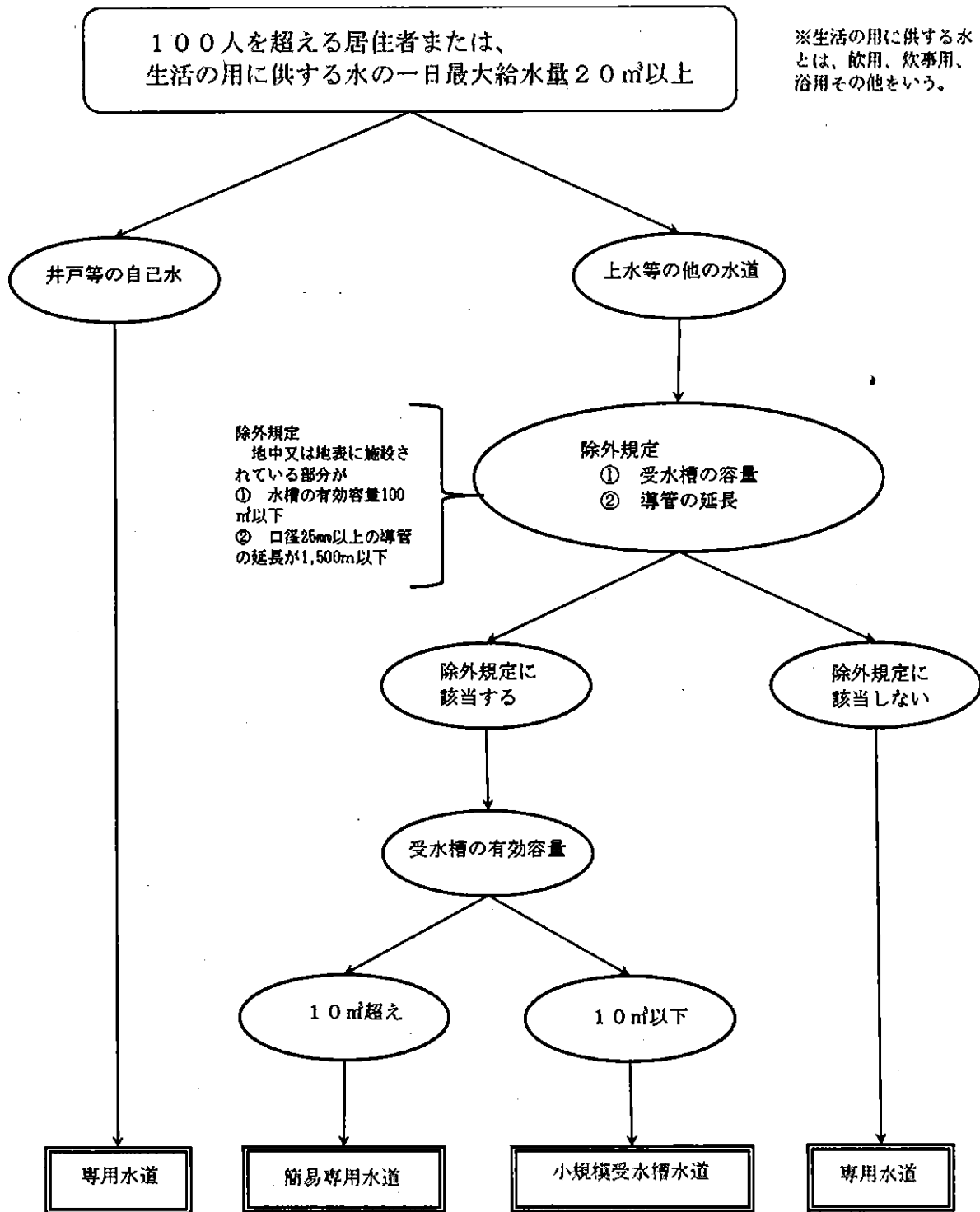
図2-7 貯水槽水道フロー図
