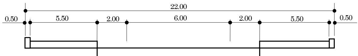
3・4・4 1 4 花川南 5 条通（橋梁部） （2 2 m、2 車線）
