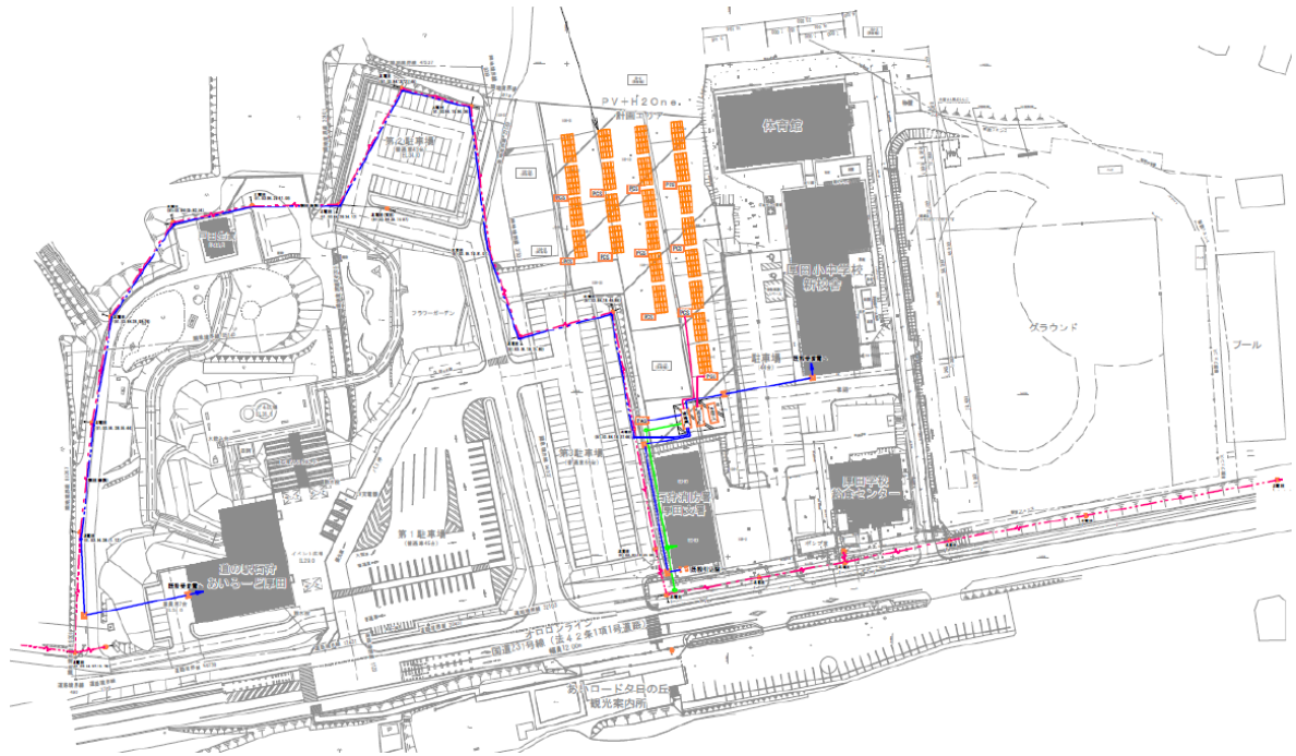
図4.1 事業対象用地
